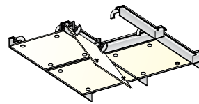
Abklappbare Variante mit punktgehaltenem Glas Fold-Out system with point- load-fixing of the glass
