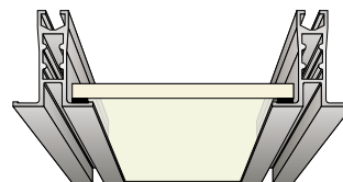
P-AL 204 mit eingelegtem Glas with Glass Inlay
