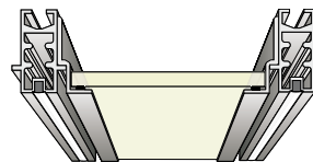
P-AL-301 mit eingelegtem Glas with Glass Inlay
