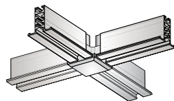
P-AL 200 mit sichtbarem Knotenpunkt KN-AL 700 Visible Joint
